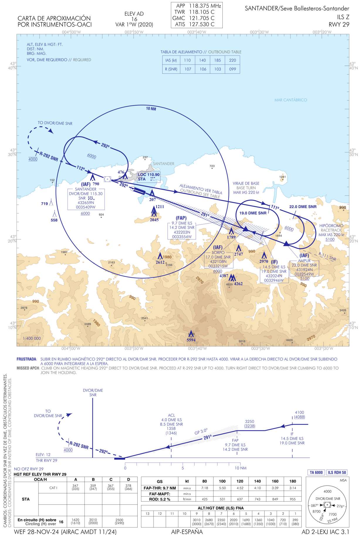
Figura 3.26: Aproximación por instrumentos a LEXJ RWY 29 procedimiento ILS [Fig31].
